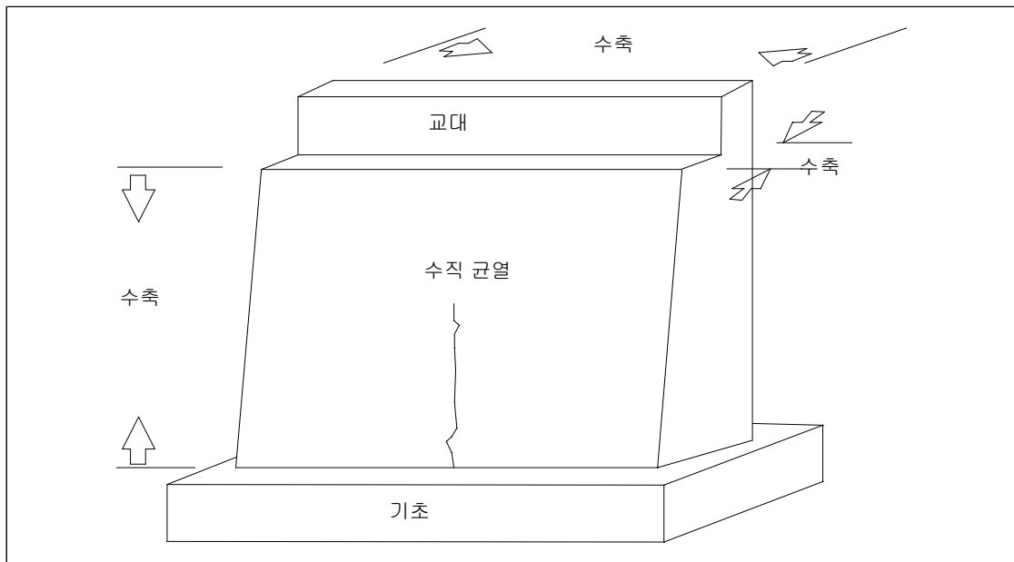
【그림 3.2.7】 온도응력, 전조수축에 의한 교대의 수직균열
